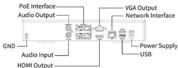
[NVR-104B-P4]
